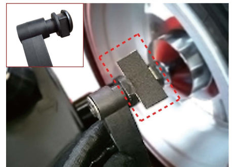
ディスタンスバー先端 貼付けウエイトクリップ付
